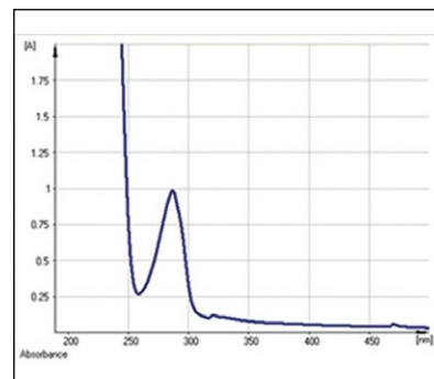
Рисунок 6. Электронный спектр кривой поглощения раствора катехина.
