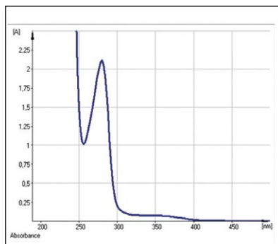
Рисунок 5. Электронный спектр кривой поглощения извлечения из плодов шиповника коричневого (г. Самара).
