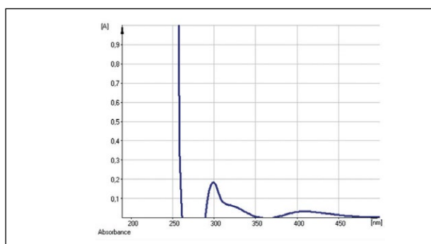
Рисунок 13. Электронный спектр дифференциальной кривой поглощения из шиповника коричневого (Республика Марий Эл).
